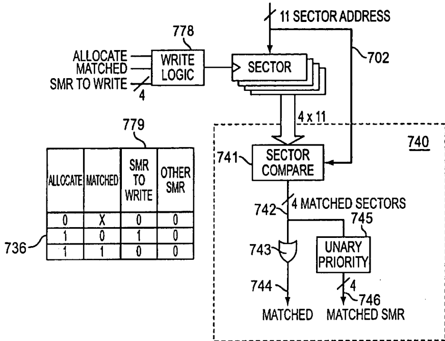
Sector match logic FIG. 7E
